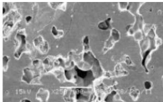
Gambar 3. Scanning Electron Micrograph dari Layer Pertama (100%Ti)
