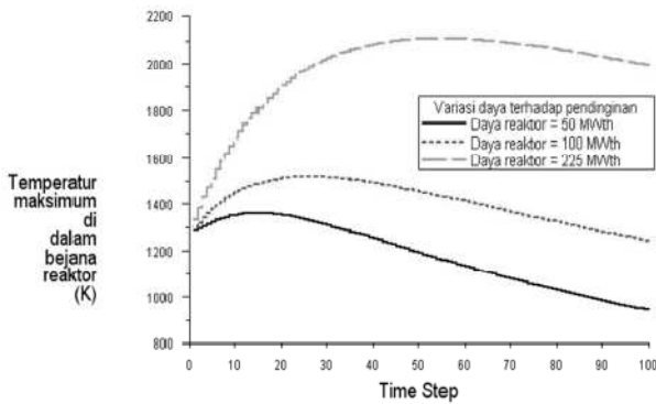
Gambar 2. Grafik perubahan suhu maksimum bahan bakar fungsi waktu dengan proses transfer panas murni konduksi pada berbagai tingkat daya reaktor.
