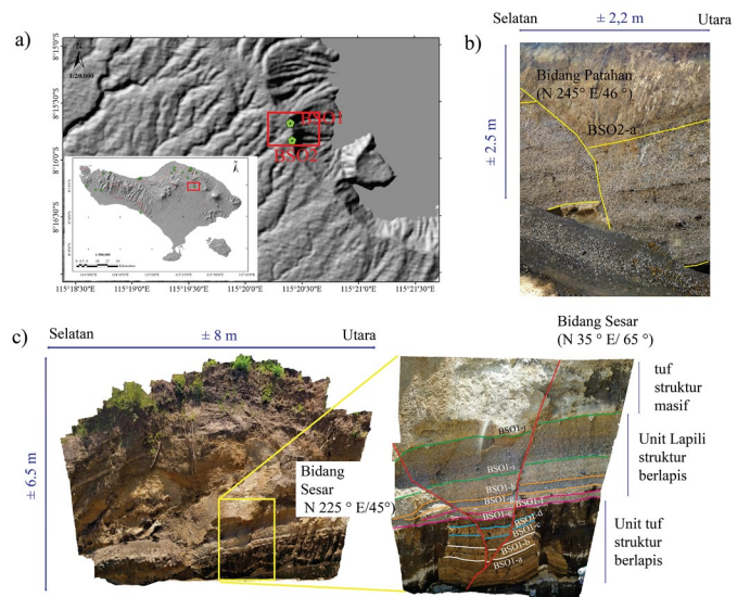
Gambar 9. Lokasi singkapan batuan (a), terdiri dari unit lapili yang tersesarkan menunjukkan komponen turun di dinding kaldera Gunung Batur di lokasi BS02 (b) dan unit tuf yang tersesarkan membentuk graben kecil di lokasi BS01 (c).
