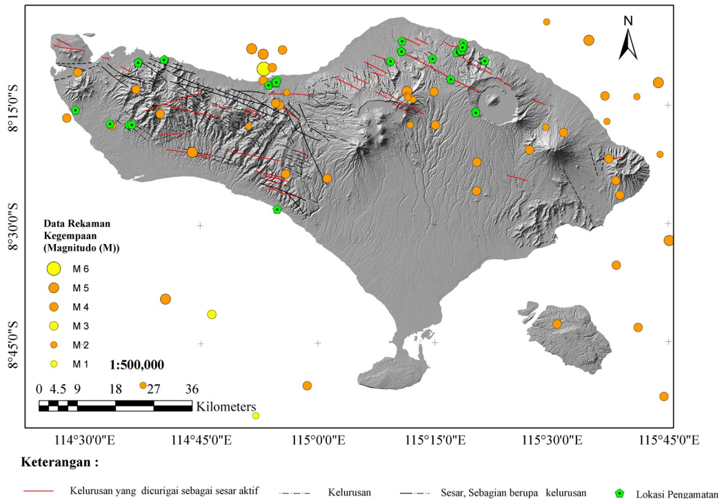
Gambar 2. Peta menunjukkan sebaran rekaman kegempaan Pulau Bali pada rentang tahun 1963-2020 (Katalog USGS, https://earthquake.usgs.gov/earthquakes/search ) dan hasil analisis kelurusan Pulau Bali yang teridentifikasi sebanyak 31 kelurusan yang dicurigai sebagai jalur sesar aktif. Orientasi kelurusan didominasi oleh kelurusan yang berarah relatif BL-TG dan sebagian kecil berarah Timur Laut –Baratdaya (BD-TL)
