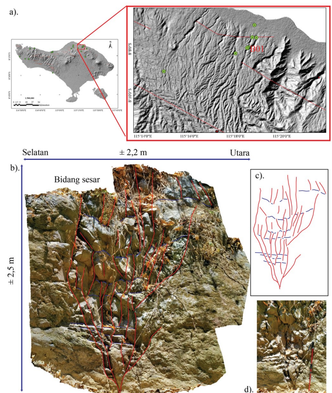
Gambar 7. Menunjukkan lokasi singkapan batuan dengan kode B01 (a) dan Zona sesar pada singkapan lava dengan geometri berbentuk bunga mekar mini ( flower structure ) yang diinterpretasi sebagai bagian paling ujung dari struktur sesar geser (b, c dan d)
