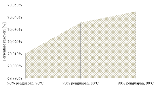
GAMBAR 4. Grafik pengaruh temperatur terhadap persentase rekovery litium
