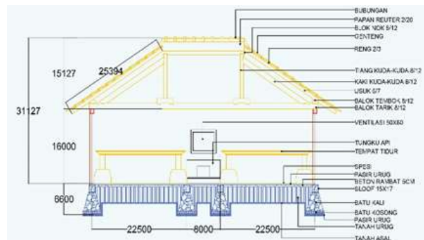
Gambar 6. Pola Ruang Dalam Rumah Di Desa Pengotan (Sumber: Analisis Pribadi,2021)
