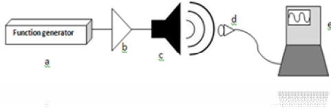
Gambar 1 Skema Kalibrasi Alat. a. Function Generator ; b. Amplifier ; c. Speaker ; d. Mikروفon; e. Komputer jinjing dilengkapi perangkat lunak Visual Analyser .
