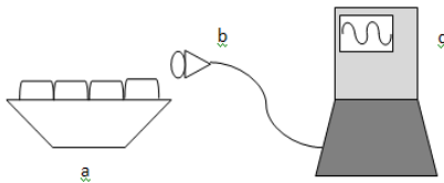
Gambar 2 Skema Percobaan pada Saron Demung. a. Saron Demung Laras Pelog; b. Mikروفon; c. Komputer jinjing dilengkapi perangkat lunak Visual Analyser
