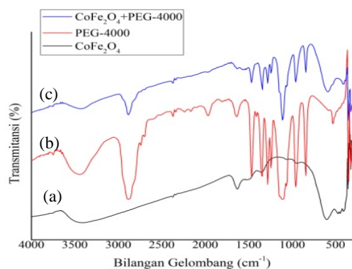
Gambar 3. Spektrum FTIR (a) CoFe 2 O 4 , (b) PEG-4000, dan (c) CoFe 2 O 4 yang dilapisi PEG-4000.
