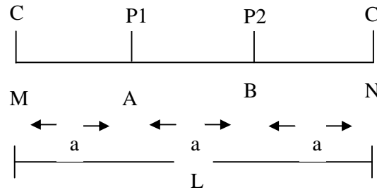
Gambar 1. Elektroda arus dan potensial pada konfigurasi Wenner.
