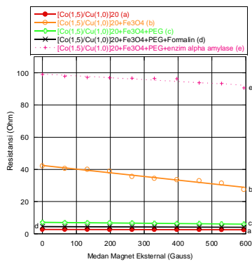
Gambar 14. Hubungan R dengan H pada lapisan tipis (a) [Co(1,5)/Cu(1,0)]_{20} multilayer dengan pelapisan nanopartikel (b) Fe_3O_4 , (c) Fe_3O_4 +PEG, (d) Fe_3O_4 +PEG+Formalin, dan (e) Fe_3O_4 +PEG+ \alpha -amylase.
