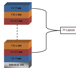
Gambar 1. Struktur GMR lapisan tipis [Co(1,5nm)/Cu(x)] 20 multilayer .
