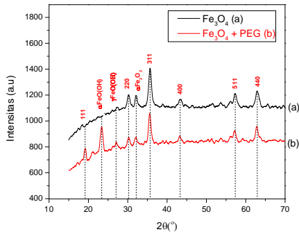
Gambar 3. Pola spektrum XRD (a) Fe_3O_4 dan (b) Fe_3O_4 yang dengan dienkapsulasi dengan PEG.
