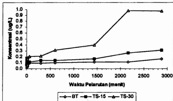
Gambar 4. Pengaruh waktu pengadukan terhadap Pb
