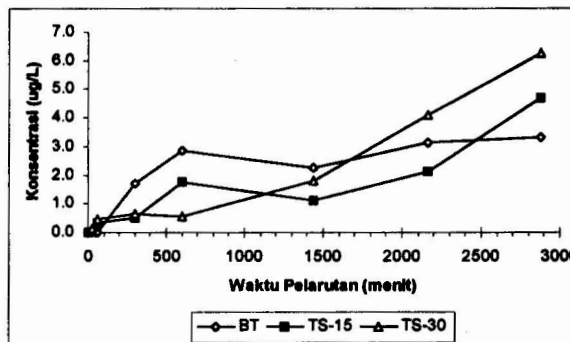
Gambar 5. Hasil analisis Zn pada berbagai konsentrasi salinitas
