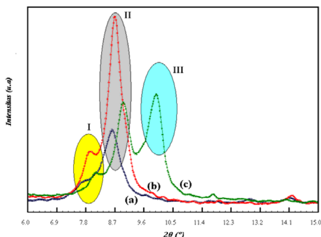
Gambar 5. Pola difraksi sinar-X pada bidang (200) spesies polikation Zr(IV) tetrahidroksida pada berbagai pH lingkungan reaksi: (a). 0,1; (b). 0,9 dan (c). 1,8
