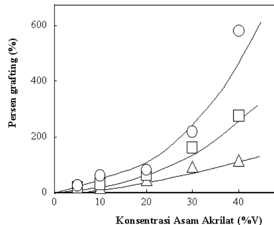
Gambar 2. Pengaruh konsentrasi monomer pada grafting asam akrilat ke polietilen yang diradiasi pada dosis 15 kGy dengan sinar- \gamma selama (○) 1 jam, (□) 2 jam dan (△) 3 jam. Suhu polimerisasi: 65°C.
