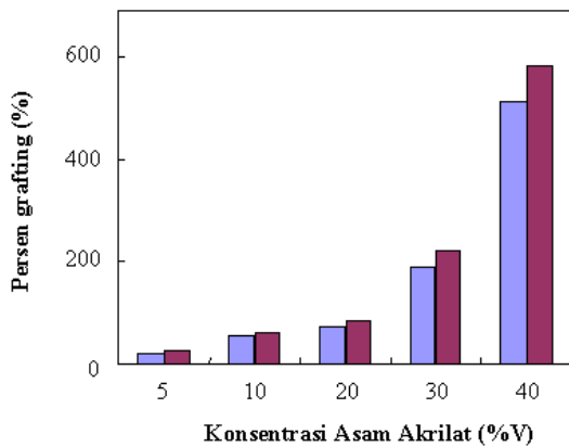
Gambar 4. Pengaruh pelarut metanol pada grafting AA ke Film PE yang telah diradiasi sinar-g. Suhu polimerisasi 65°C, 3 jam.
