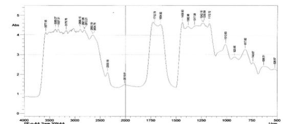
Gambar 6. Spektrum IR polietilen tergrafting asam akrilat (PE-g-AA)
