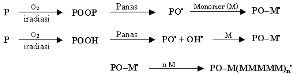
Gambar 3. Reaksi polimerisasi grafting AA pada film PE
