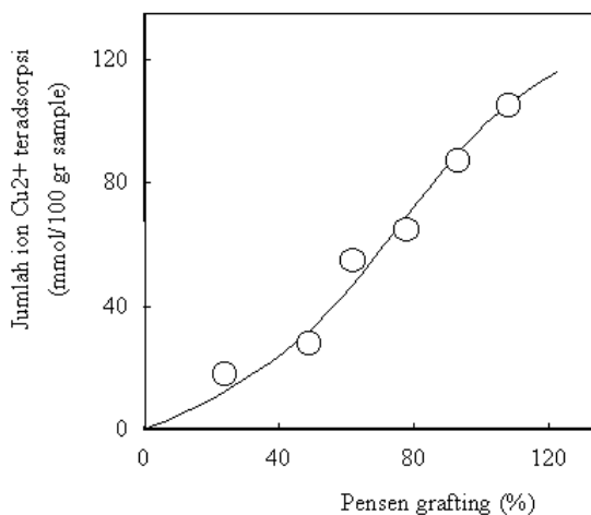
Gambar 9. Hubungan antara jumlah ion \text{Cu}^{2+} teradsorpsi dengan persen grafting AA tergrafting film PE. (25°C, 24 jam, [\text{Cu}^{2+}] = 1,79 \times 10^{-2} mol/l).
