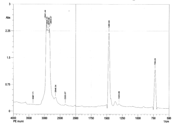
Gambar 5. Spektrum IR polietilen murni
