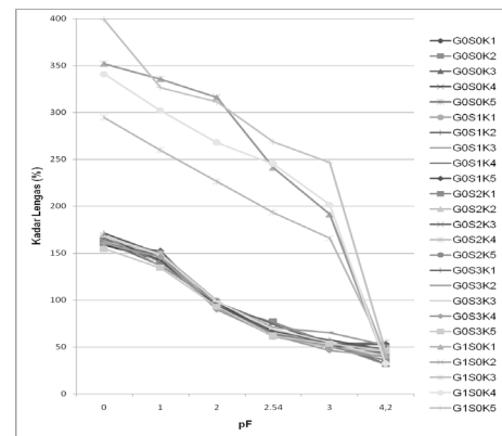
Gambar 2. Kurva tegangan lengas (pF 0 sampai 4,2)
