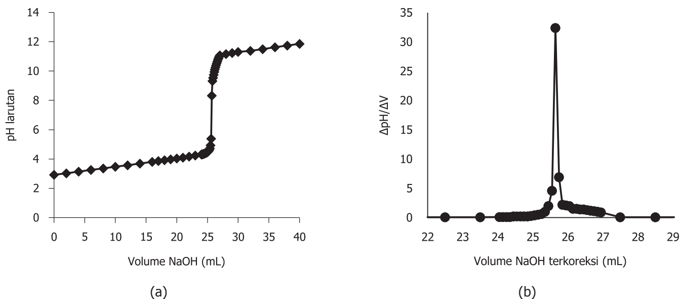
Gambar 3. Kurva titrasi CH 3 COOH dengan NaOH (a) hubungan antara pH dengan volume titran, (b) kurva turunan pertama
