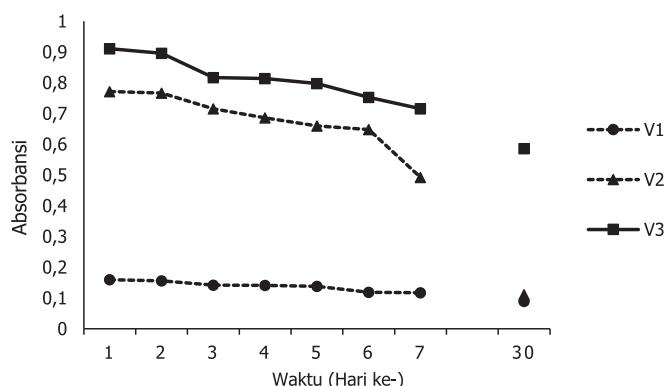
Gambar 2. Kurva absorbansi maksimal selama penyimpanan. V1: variasi pelarut 1, V2: variasi pelarut 2, dan V3: variasi pelarut 3
