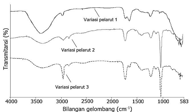
Gambar 1. Spektrogram inframerah ekstrak pekat kulit buah naga dari 3 variasi pelarut
