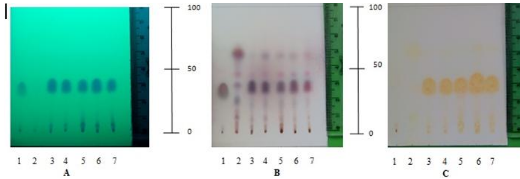
Gambar 1. Profil Kromatogram Minyak Kombinasi dan Hasil Ekstraksi Granul
