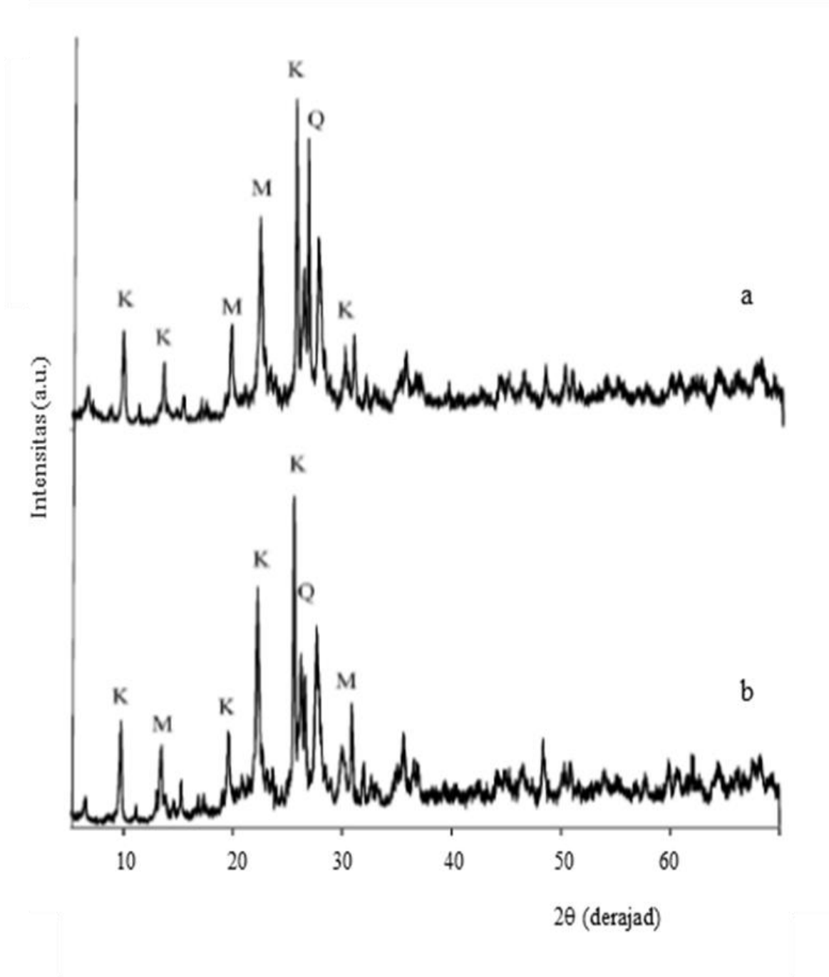
Gambar 3. Difraktogram sinar-X sampel (a) zeolit termodifikasi propilamin dan (b) zeolit termodifikasi CTAB. Keterangan: K = klinoptilolit, M= mordernit, Q= kuarsa
